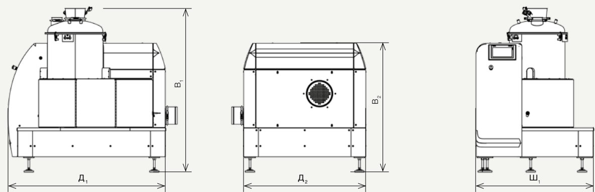
Вид спереди
