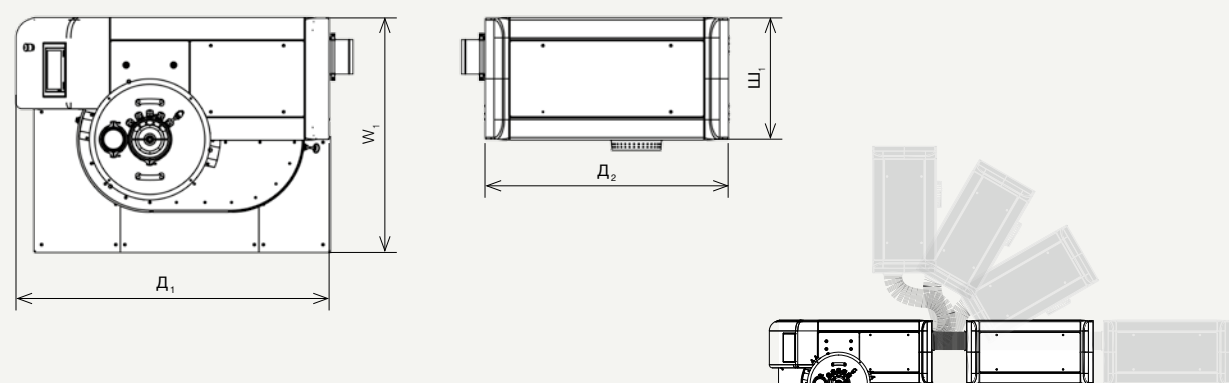
Вид сверху
